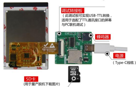
图 1-5 调试工具图
