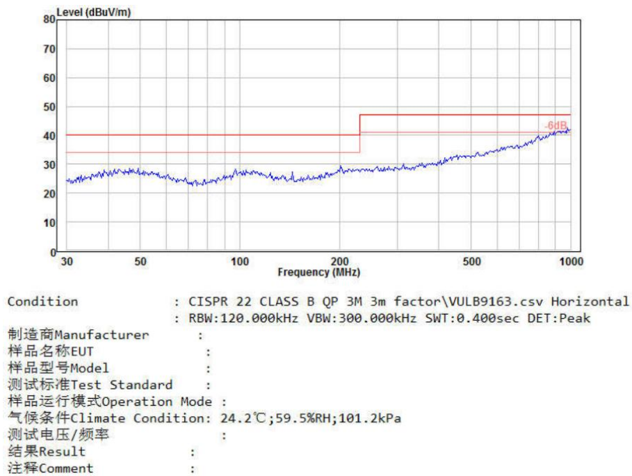
图 6-5 RE 测试水平方向
